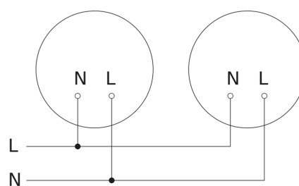
aansluitschema master/master
